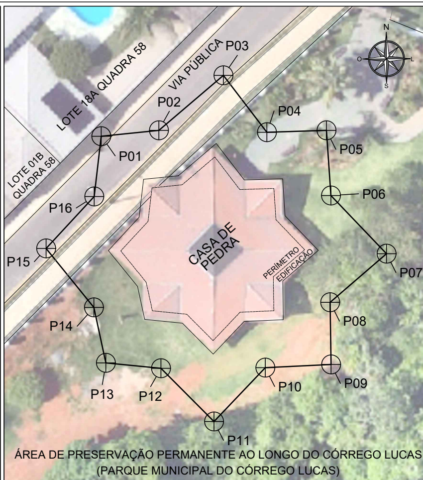
2 LOCAÇÃO ESCALA 1: 500
